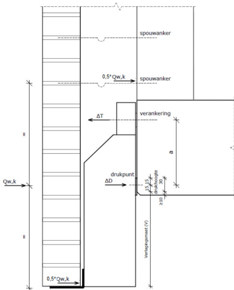
Figuur C3 – Bepalen additionele krachten t.g.v. windbelasting op metselwerk
